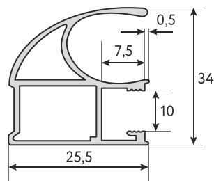
Ручка асимметричная эконом
