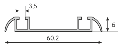
Направляющая нижняя двойная
